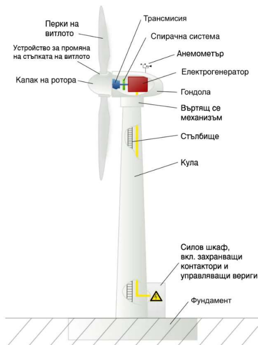
Фигура 1.2.1-1. Елементи на вятърните генератори
