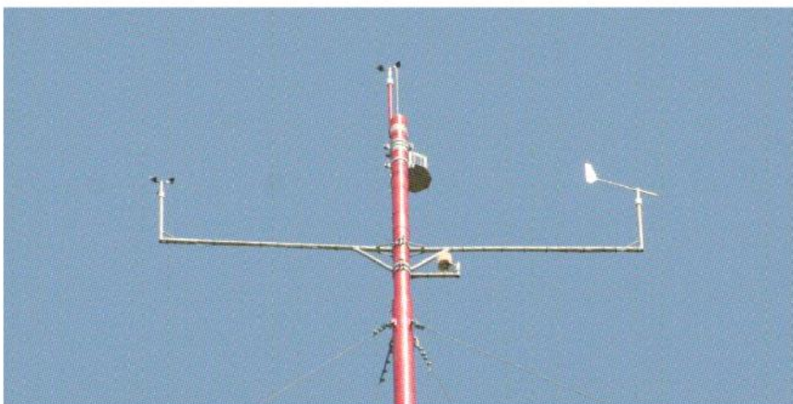
Фигура 3.1.1-2. Сензори на върха на мачтата, 100 m над земната повърхност
