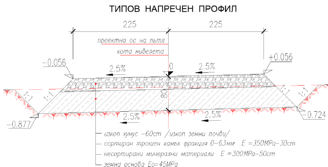
Фигура. 1.2.1-1. Типов напречен профил на пътища
